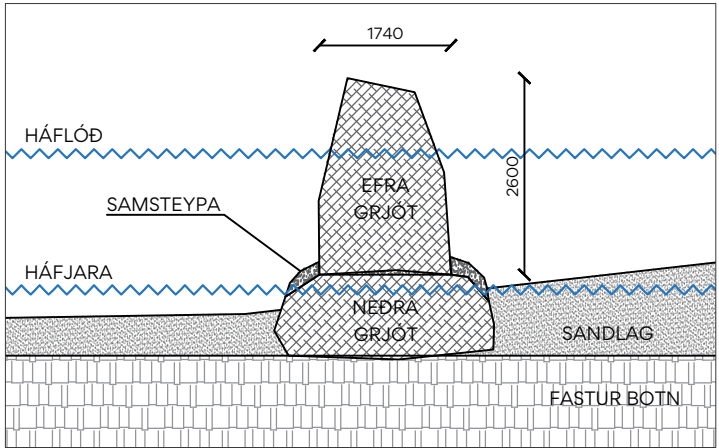
SKÝRINGASNIÐ, 1:100@A3
